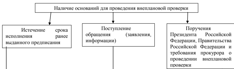
Блок-схема № 2 осуществления регионального государственного надзора за обеспечением сохранности автомобильных дорог регионального и межмуниципального значения (проведение внеплановых проверок)
